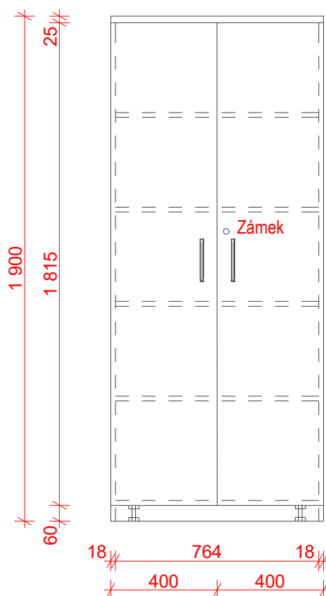
Čelní pohled
