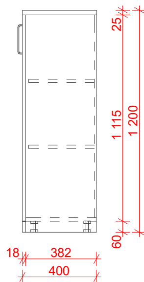
Boční pohled
