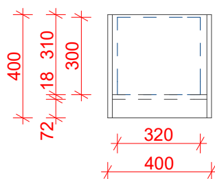
Boční pohled
