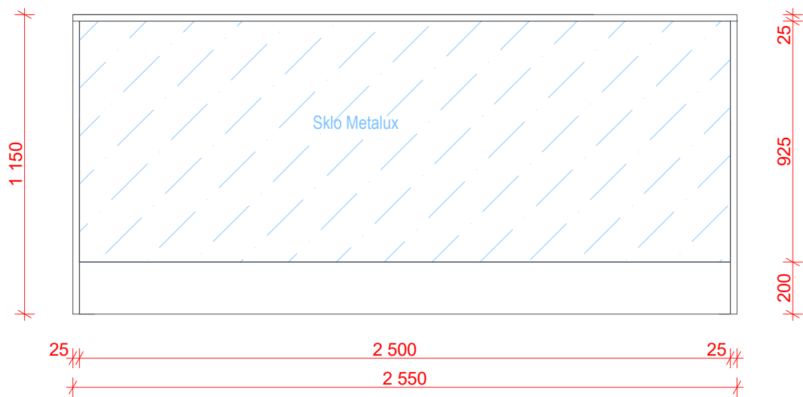
Čelní pohled
