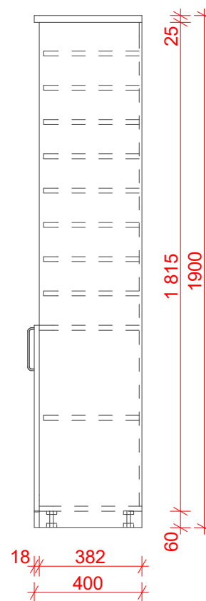
Boční pohled
