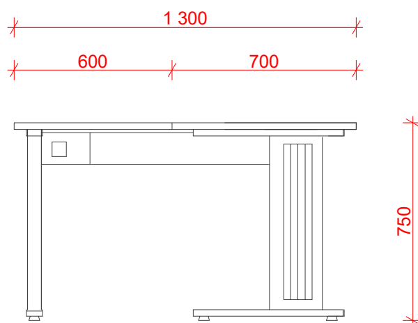
Boční pohled
