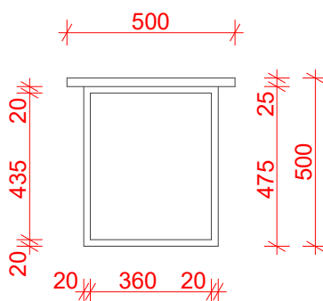
Boční pohled
