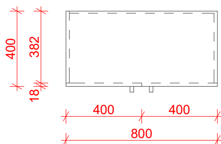
Půdorys
