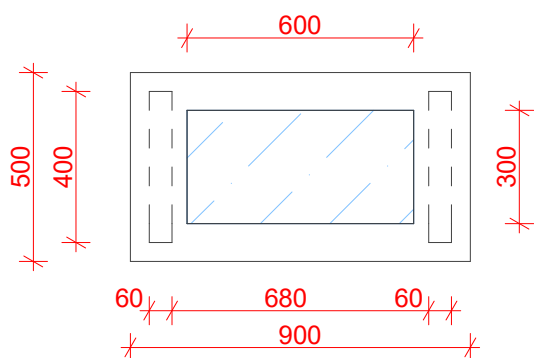
Boční pohled
