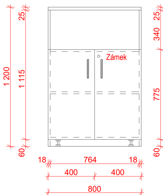
Čelní pohled
