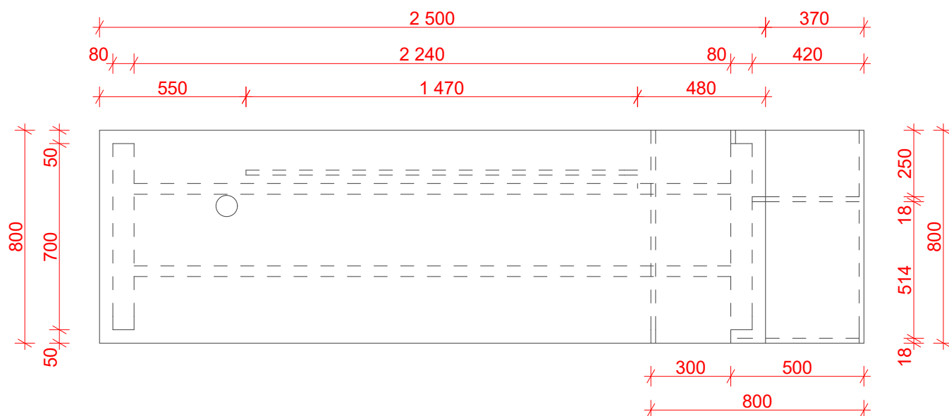
Půdorys
