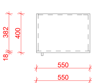
Půdorys
