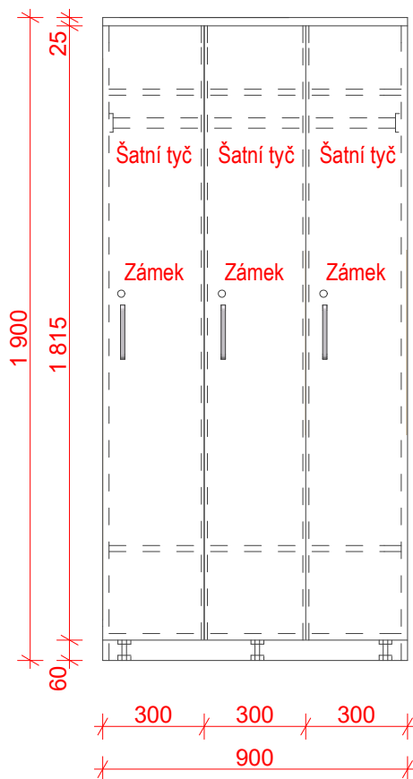
Čelní pohled
