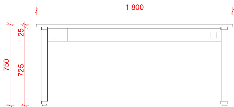
Čelní pohled
