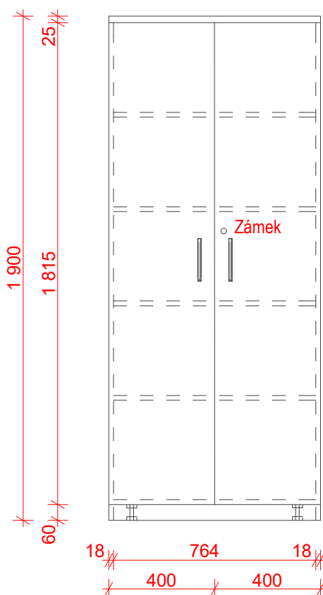
Čelní pohled
