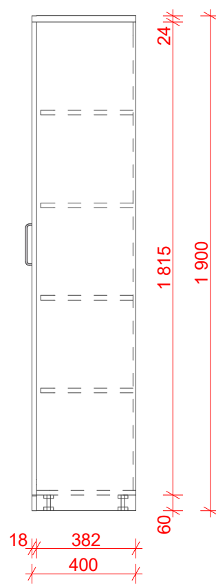
Boční pohled
