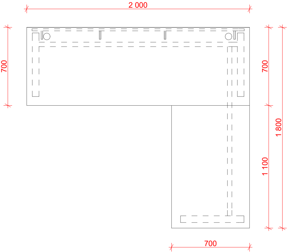
Půdorys
