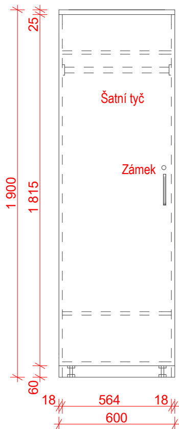
Čelní pohled
