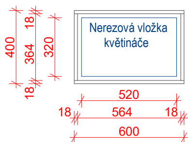
Půdorys
