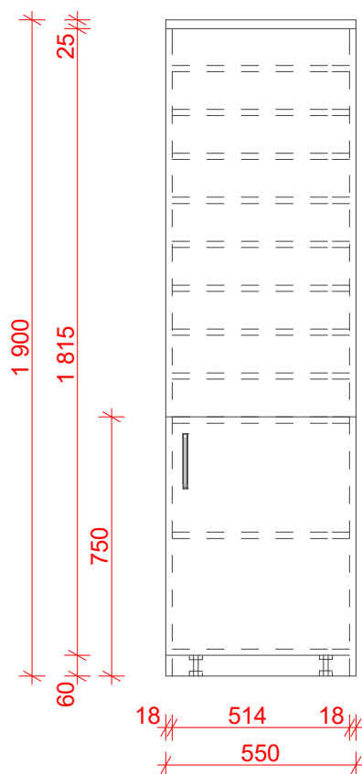
Čelní pohled
