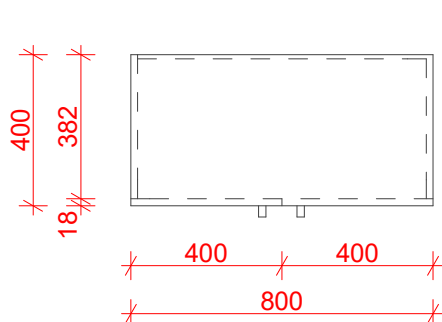
Půdorys
