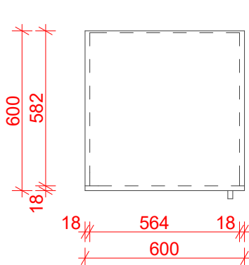
Půdorys
