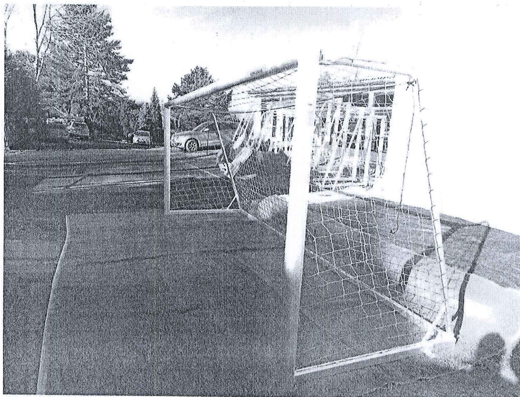
Celkový pohled na konstrukci branky č.výr.: 0255
