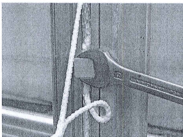
Montáž sítě pomocí úchytů
