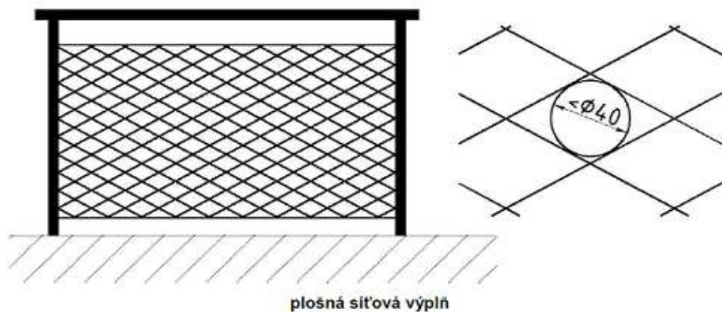
Obrázek 7 – Plošná děrovaná výplň
