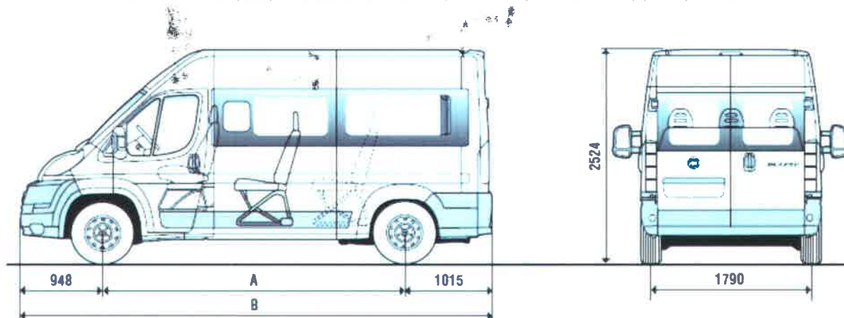
Obrázek 2 - Rozměry vozidla Fiat Ducato Combi
